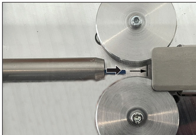
Figure 5.19 Insérer le conducteur correctement
