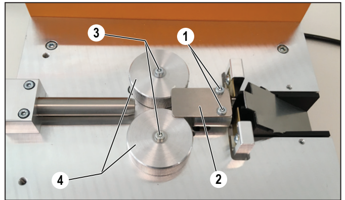
Figure 8.5 Remplacer les rouleaux d'avance
