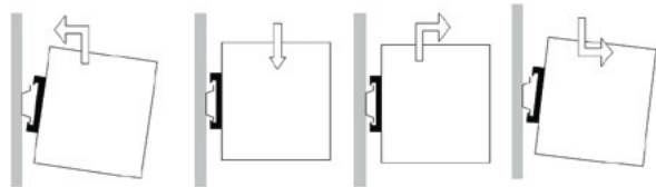
Aufrasten Snap-on
