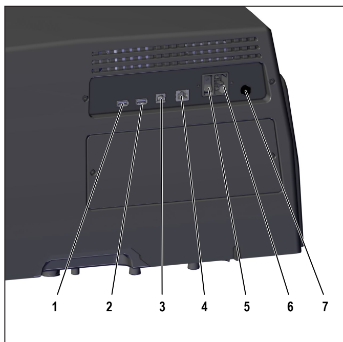
图3.4 接口
