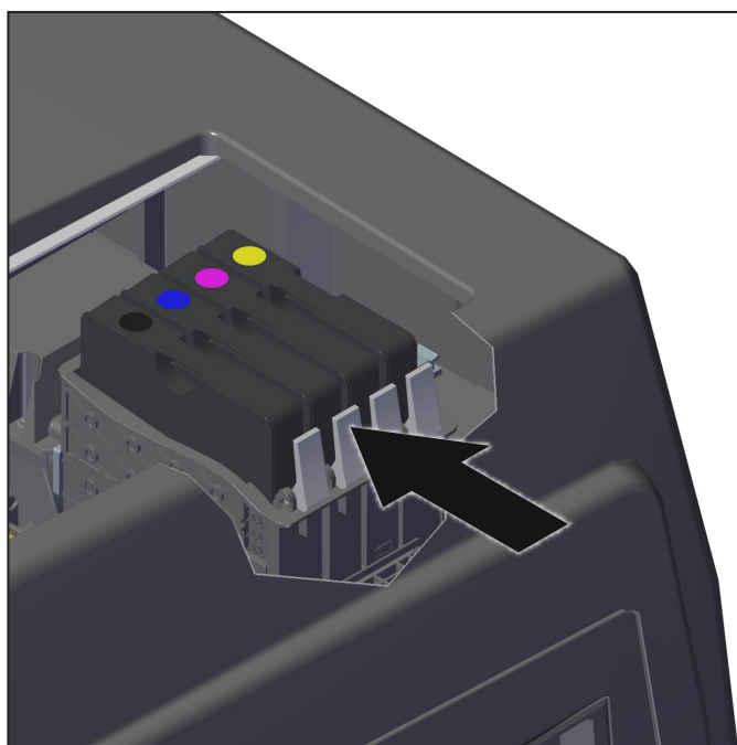
图6.12 解锁墨盒
