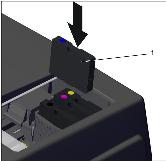
图6.14 装入墨盒
