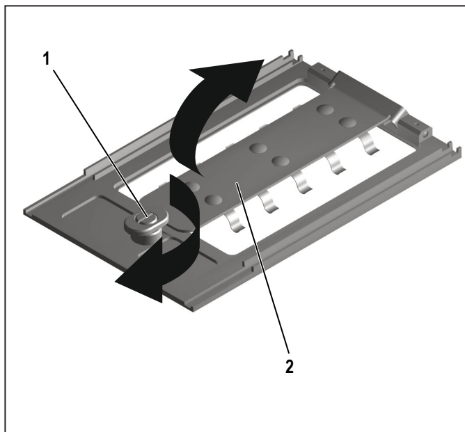
图5.2 打开嵌体
