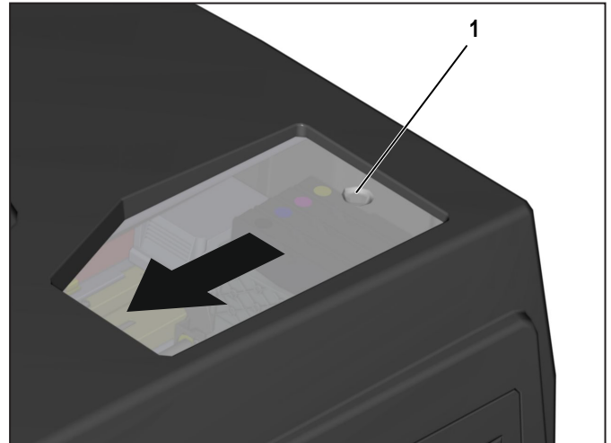
图4.9 打开墨槽盖
