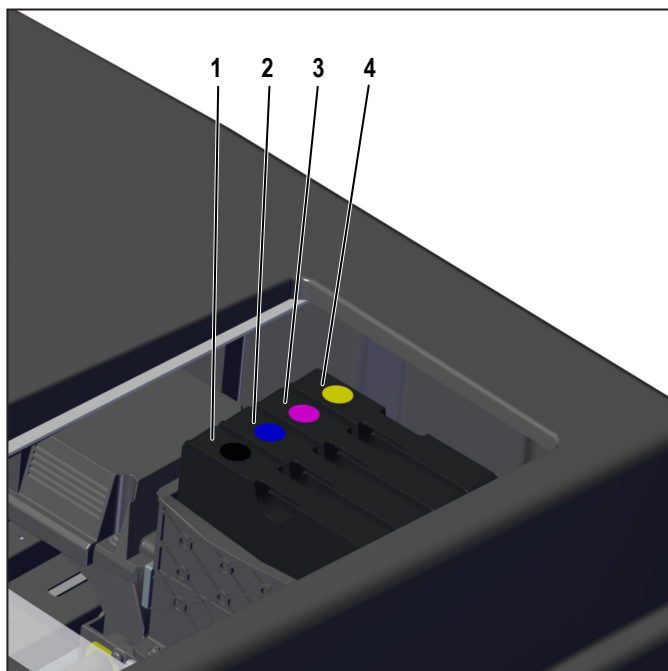
图6.11 墨盒的位置
