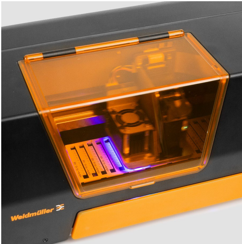
Bildunterschrift: Integrierter Druckkopf mit UV-härtender Tinte sorgt für wisch- und kratzfeste Beschriftung bei 600 dpi – in nur 90 Sekunden pro MultiCard.
