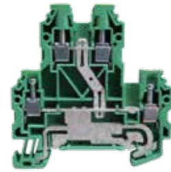
SAKDK 4N PE 4 mm 2
