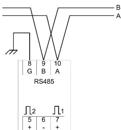
图：RS485 接口，三脚端子连接
