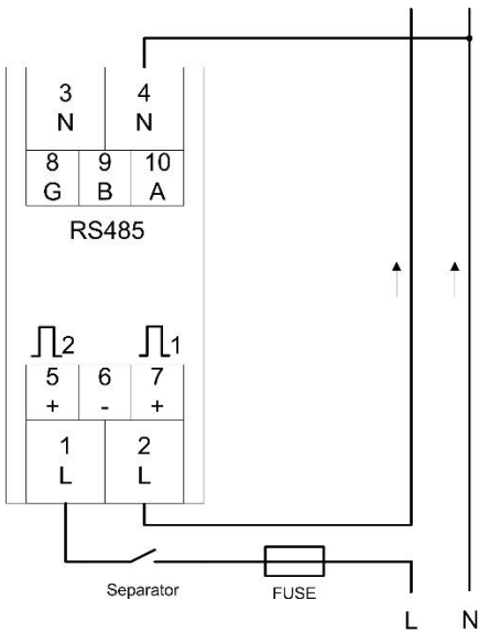
图：电压与电流测量连接示例
