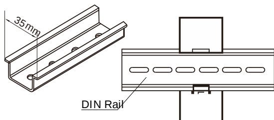
图：通过符合 DIN EN 60715 标准的导轨固定 EM111
