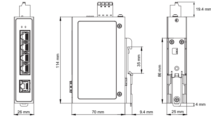
IE-SW-BLB-05-5GT IE-SW-BLB-05-5GT-C
