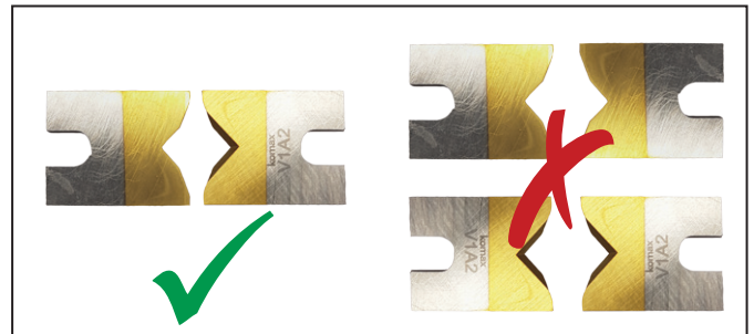
Immagine 8.2 Orientare le lame
