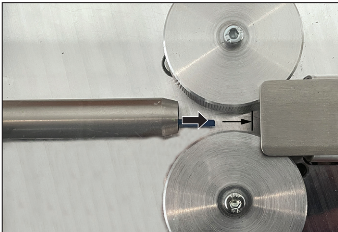
Image 6.6 Insérer le conducteur correctement
