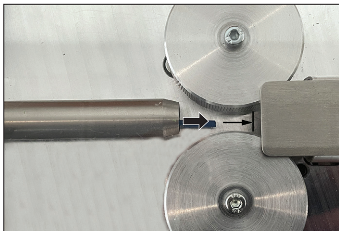
Ilustr. 6.6 Prawidłowe wprowadzanie przewodu
