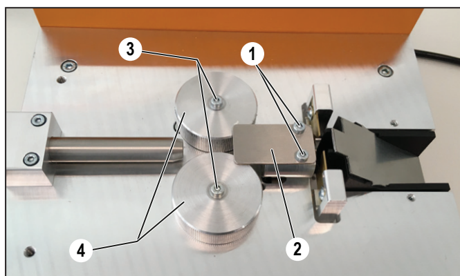
Image 8.5 Remplacer les rouleaux d'avance
