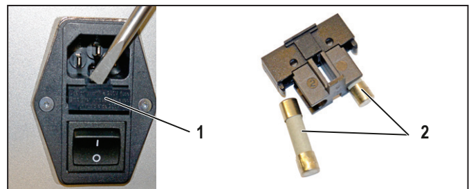
Immagine 8.3 Fusibili
