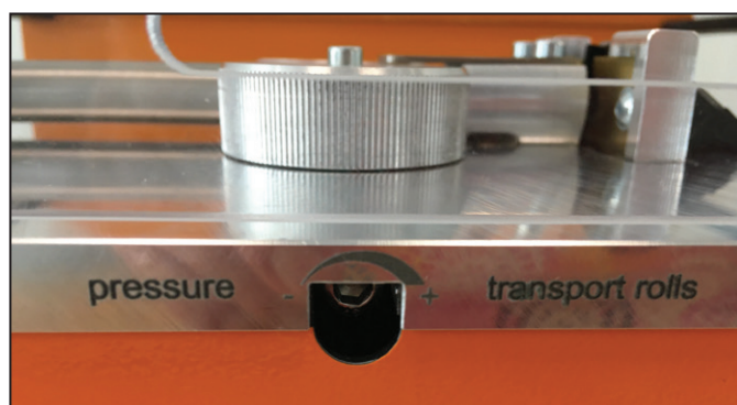
Ilustr. 8.4 Śruba nastawcza regulacji docisku
