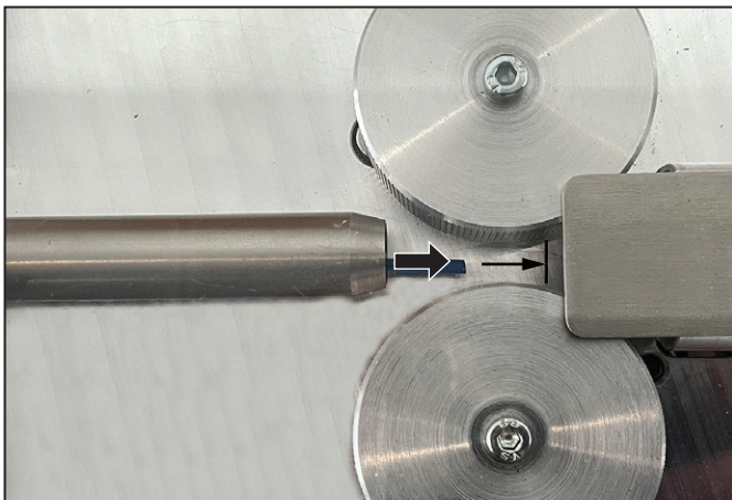
Immagine 6.6 Introdurre correttamente il conduttore
