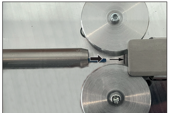
Bild 5.19 Leiter richtig einführen
