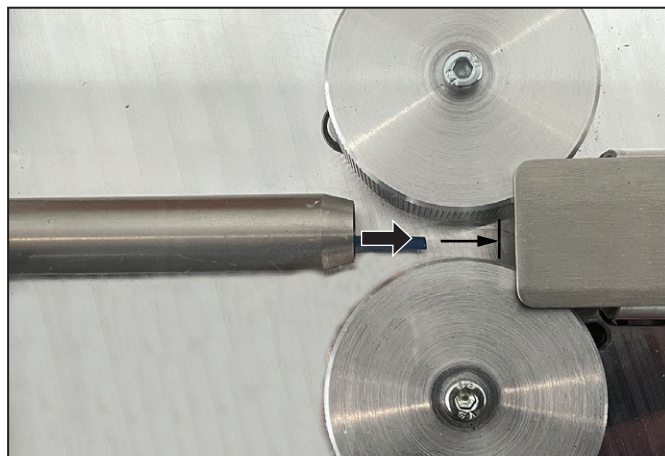
Image 5.19 Insérer le conducteur correctement
