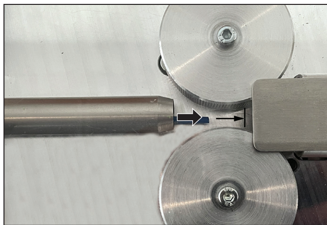
Ilustr. 5.19 Prawidłowe wprowadzanie przewodu
