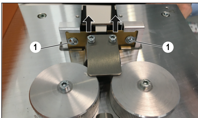
Immagine 8.1 Coltello da taglio
