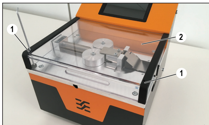
Ilustr. 7.1 Usuwanie osłony ochronnej
