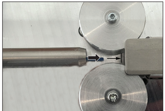
Immagine 5.19 Introdurre correttamente il conduttore
