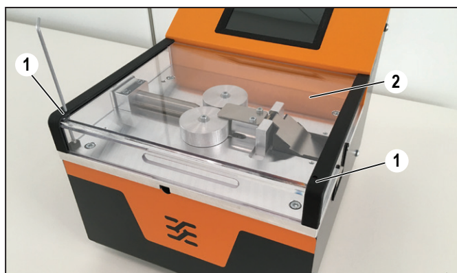
Image 7.1 Retirer le cache de protection
