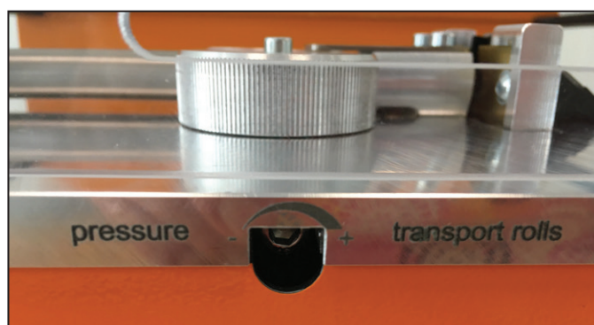
Immagine 8.4 Vite di regolazione della pressione di spinta
