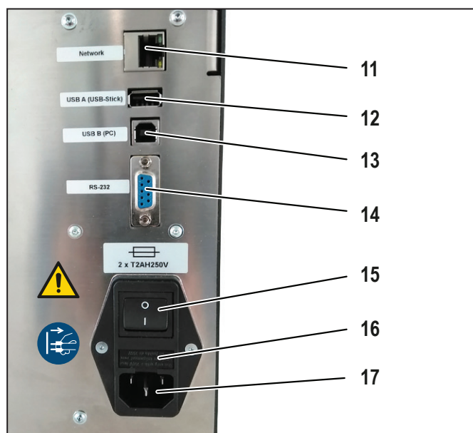
Ilustr. 3.2 Widok z tyłu
