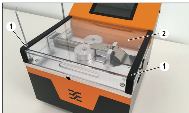
Immagine 7.1 Rimuovere la copertura di protezione
