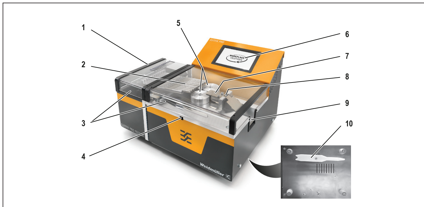
Ilustr. 3.1 Widok z przodu
