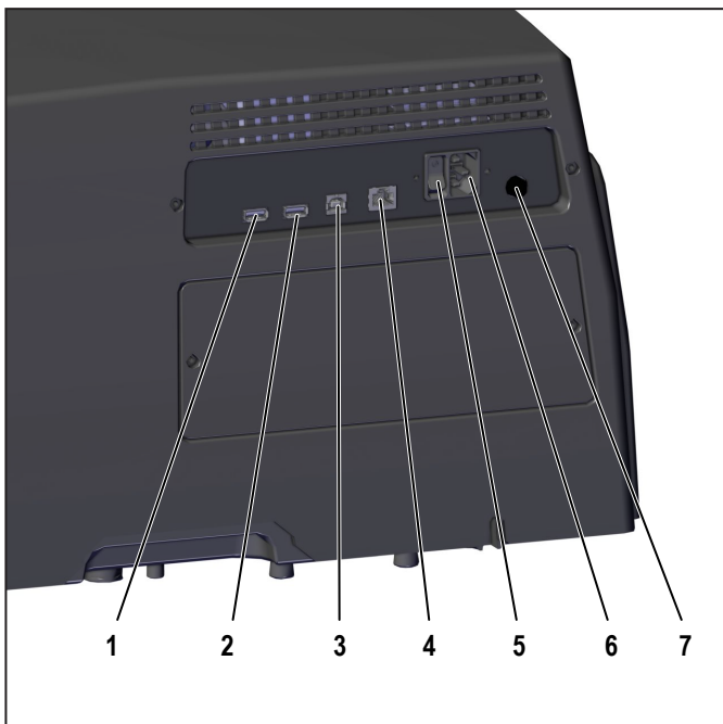
Ilustración 3.4 Conexiones
