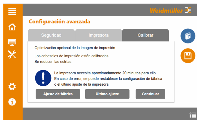
Ilustración 6.15 Menú "Calibrar"
