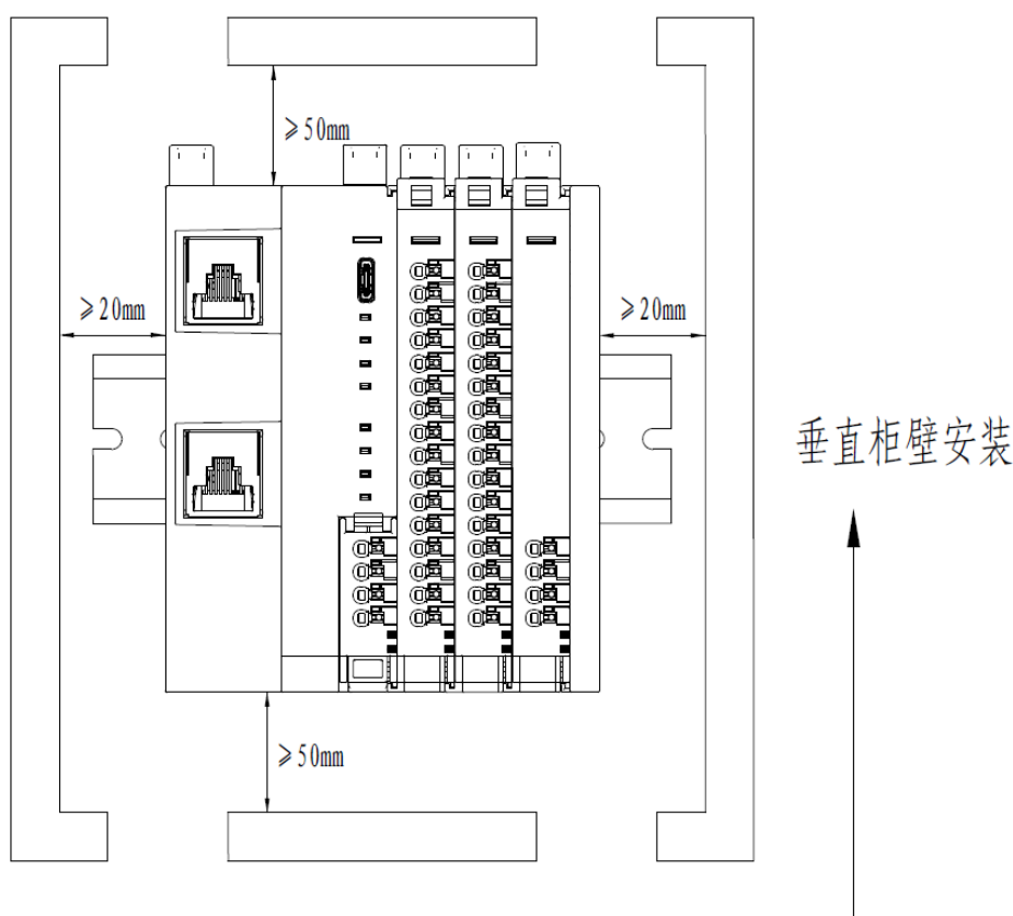
垂直柜安装示意图
